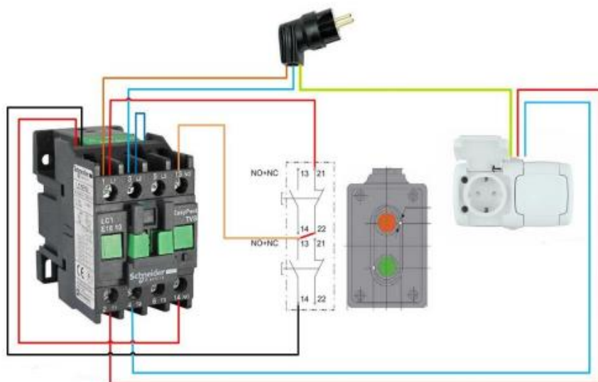
Электрическая схема подключения контактора в однофазную сеть
